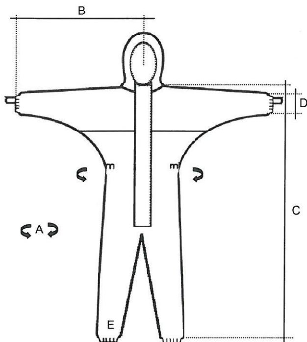
Fig. modello e dimensioni
