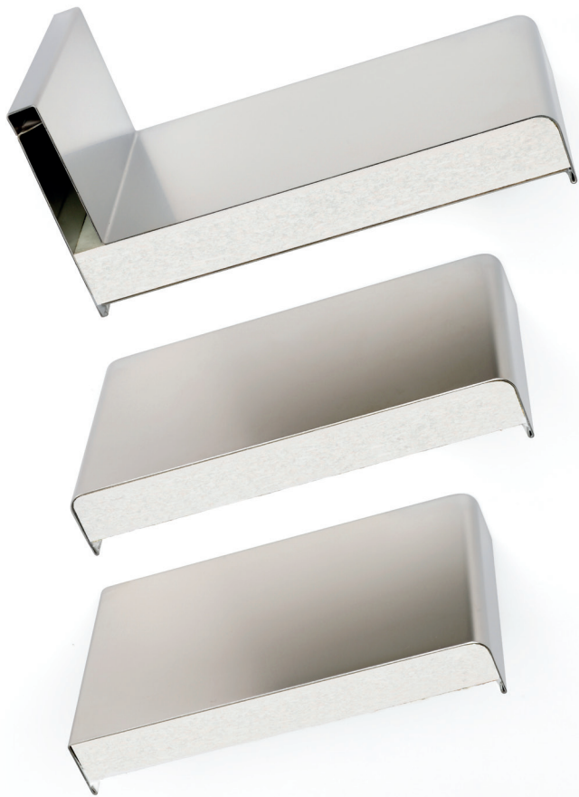
Esempi di raggiatura piani di lavoro Folding sided exemple on worktop Exemples de rayon de courbure Beispiele von Tischplatten-Radius
